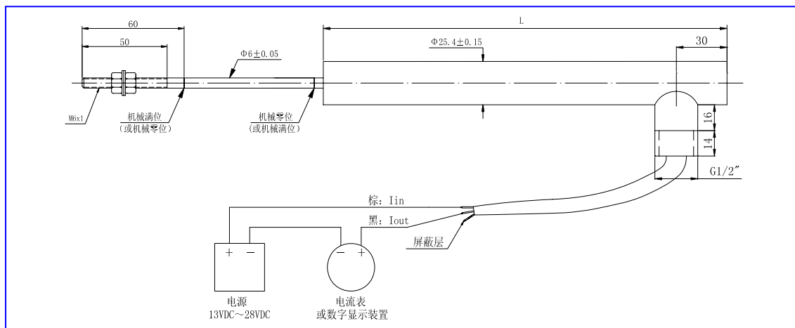
HDC2 系列位移传感器外形尺寸图
